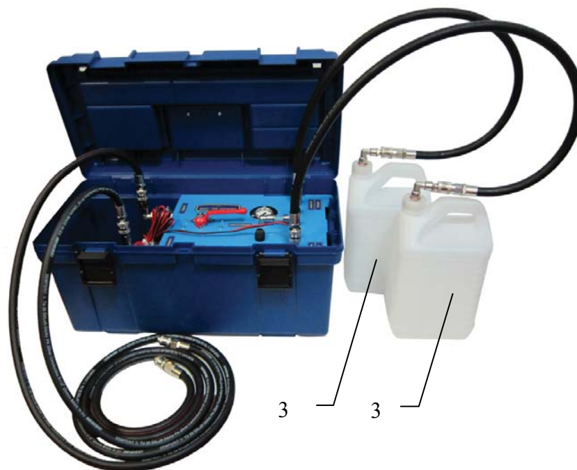
Рис.1 (вид спереди)
